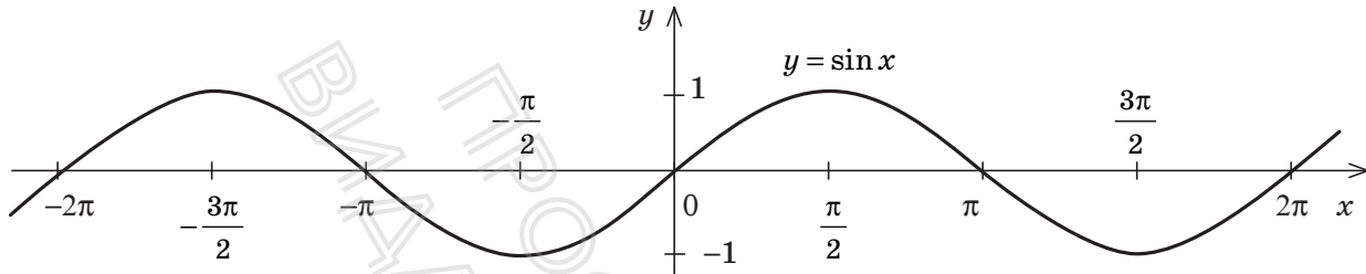
Графік функції y = \sin x (синусоїда)
